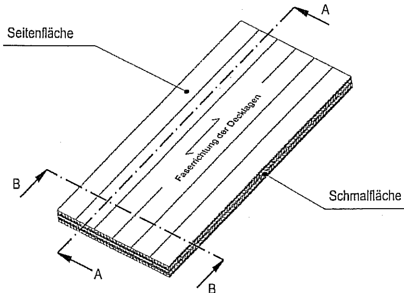
Schnitt A - A: (Darstellungen 5-lagig)
